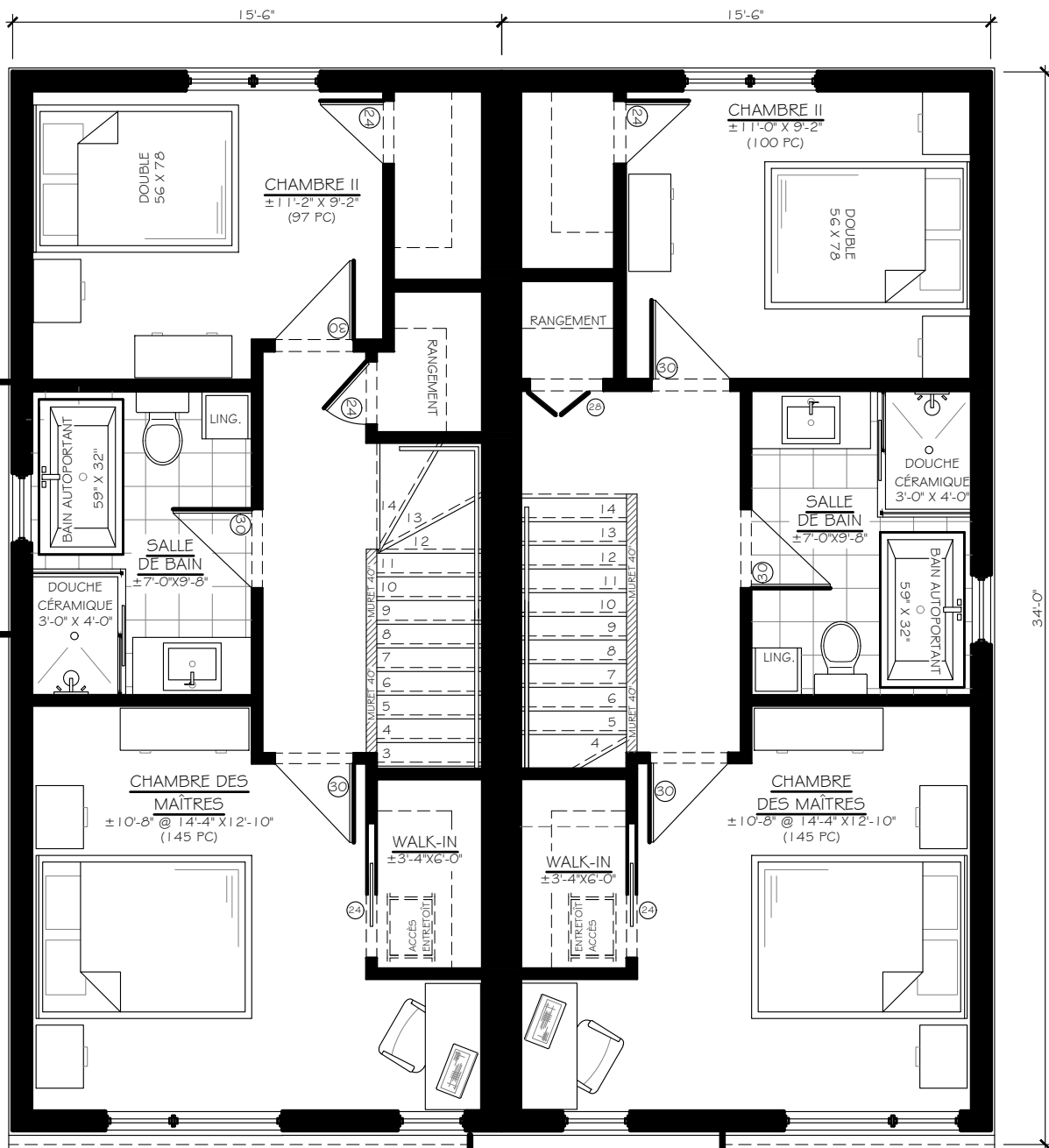
⊙ JUMLÉ 15'-6" X 34' PLAN ÉTAGE
