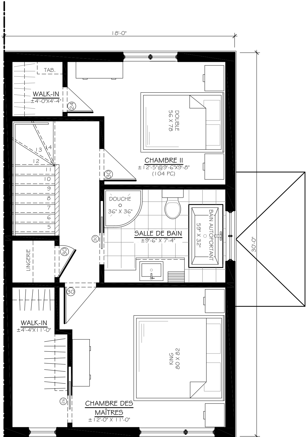
PLAN ÉTAGE COIN TARDIF SABLONNIÈRE
