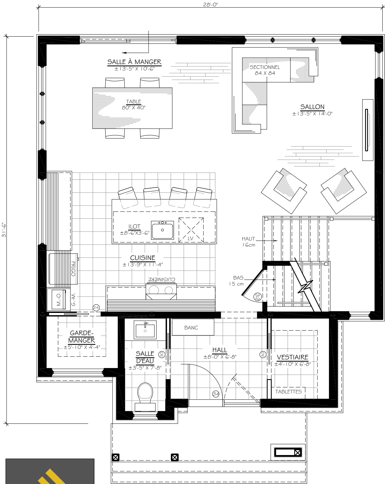
PLAN (820 pc) REZ-DE-CHAUSSÉE
