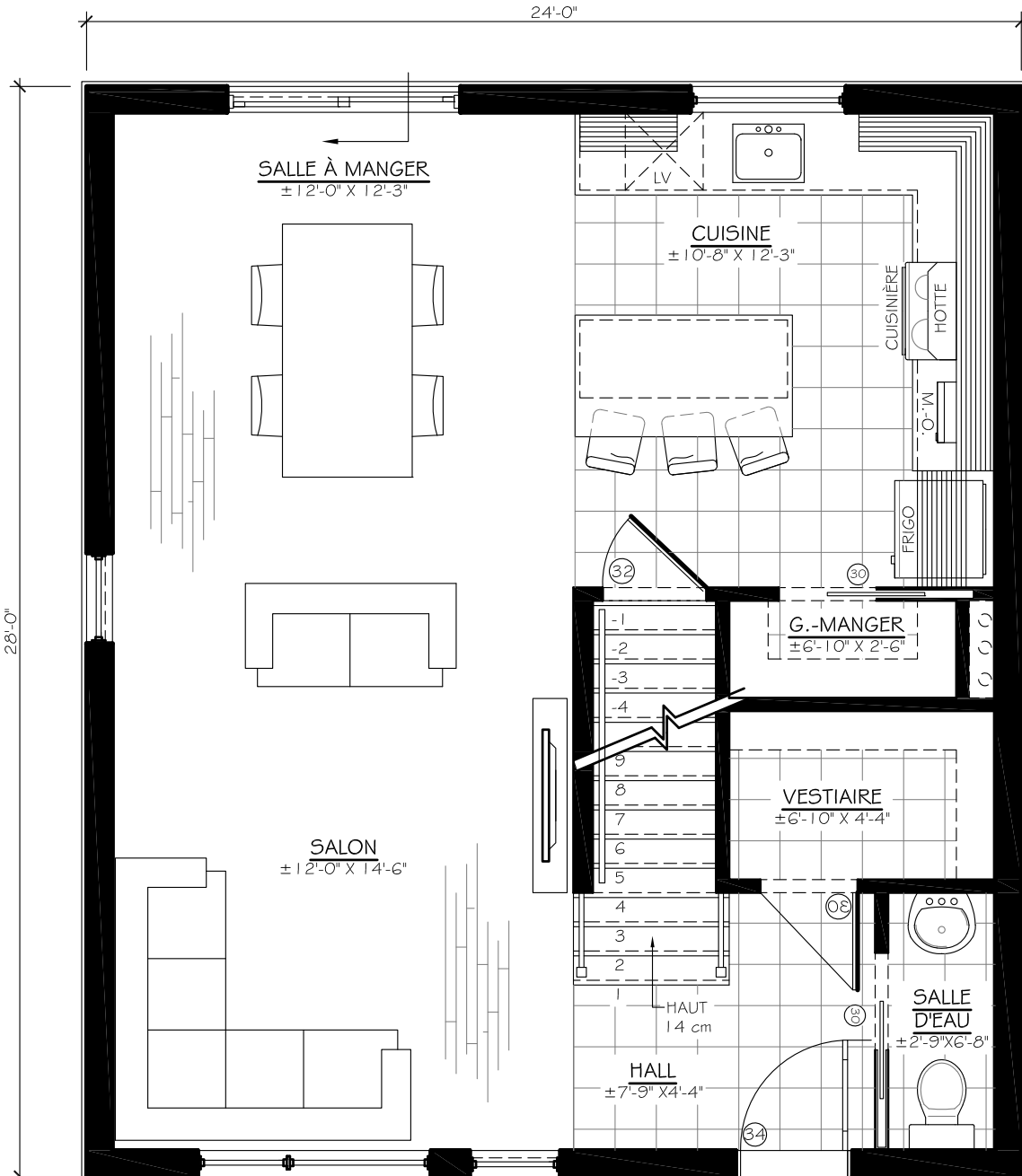
PLAN RDC
