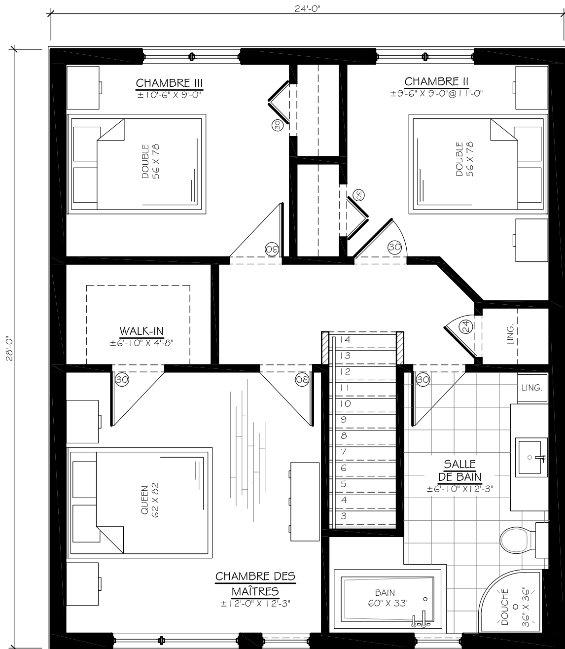
○ PLAN ÉTAGE
